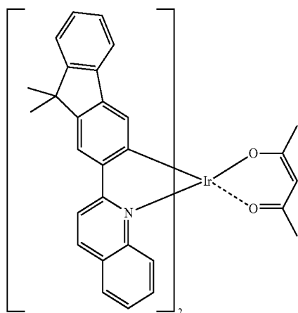
Ir(flq) 2 (acac)
