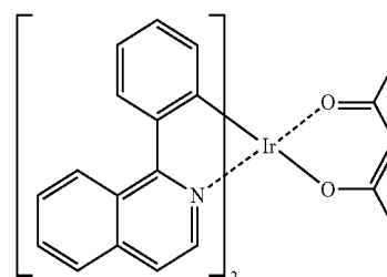
Btp 2 Ir(acac)
