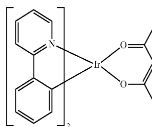
Ir(ppy) 2 (acac)
