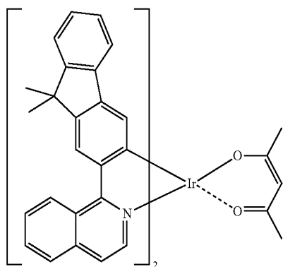
Ir(fliq) 2 (acac)
