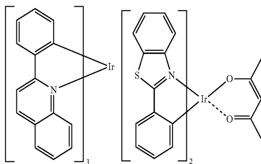
Ir(2-phq) 3
